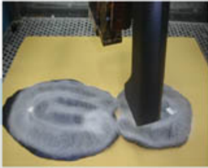
螺旋狀噴霧噴在橡膠大底
